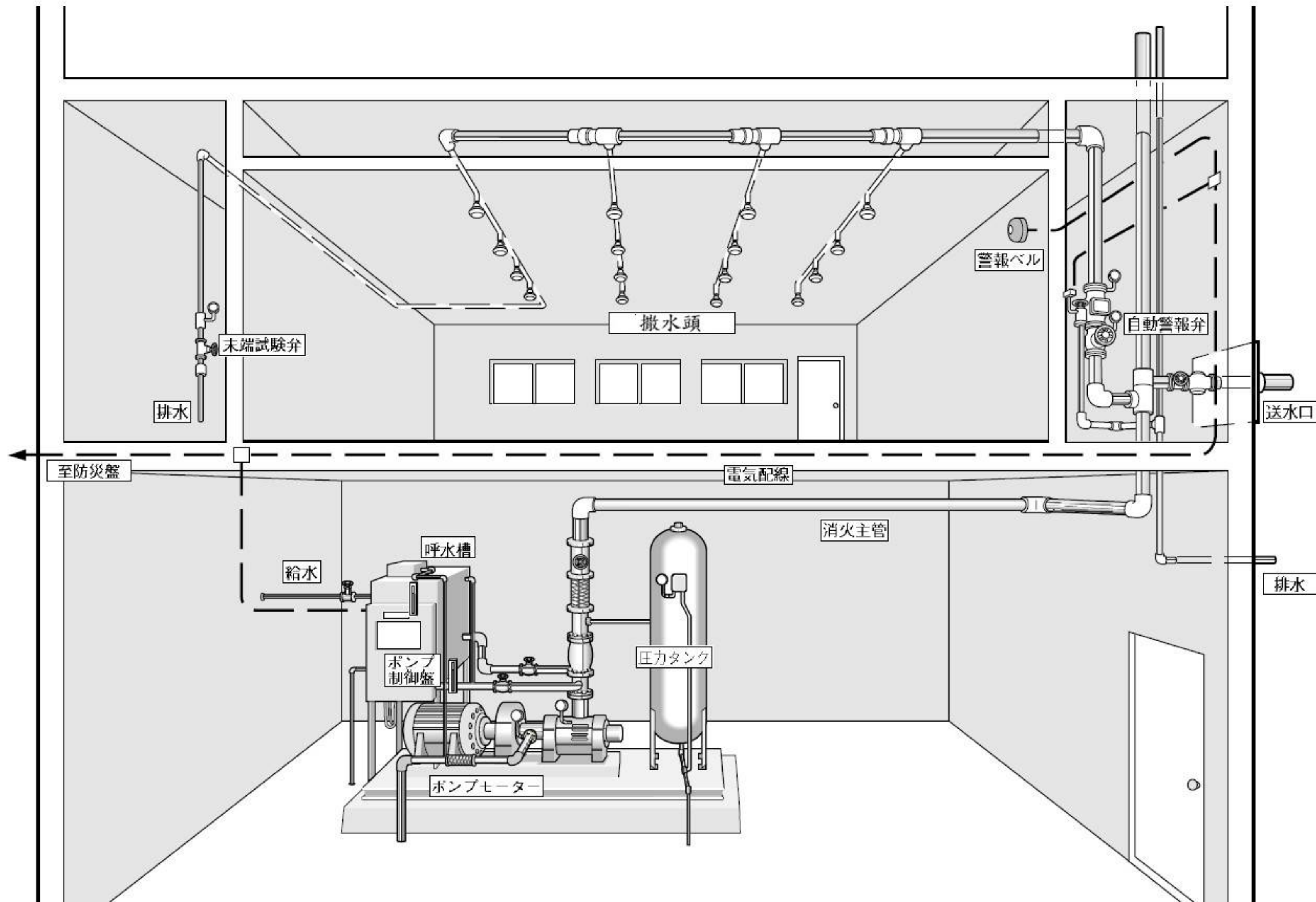
撒水系統圖
