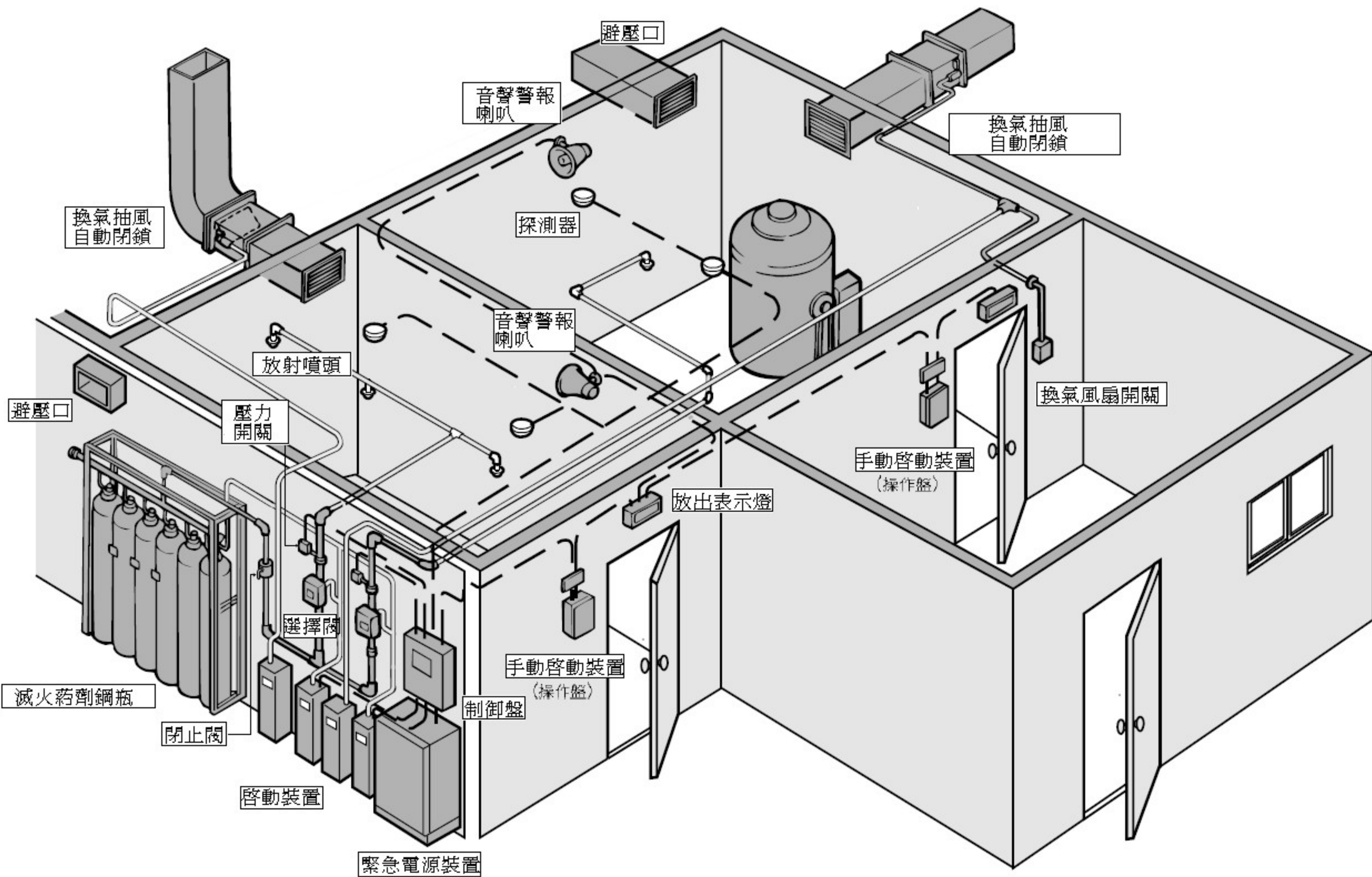
系統概念圖(集中配管式)
